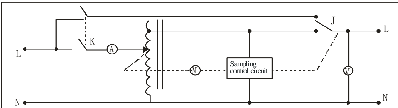
Рисунок 3: Принципиальная схема модели СН-93020 и СН-93030.
