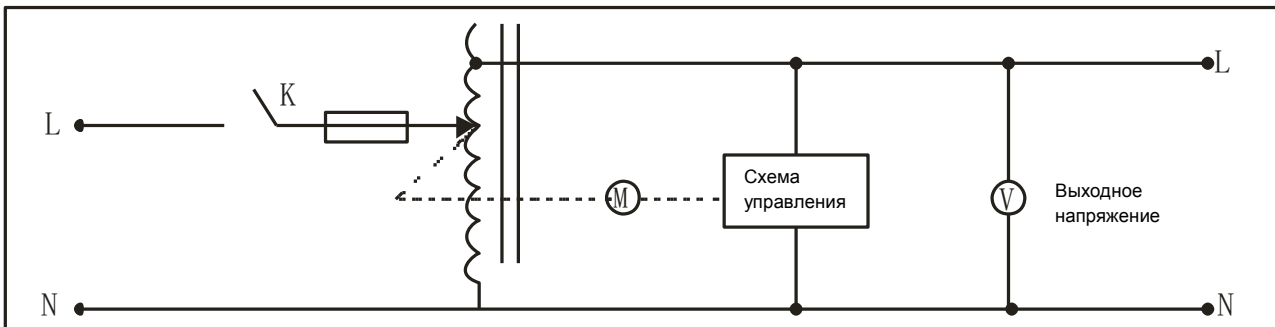
Рисунок 2: Принципиальная схема модели СН-93010.
