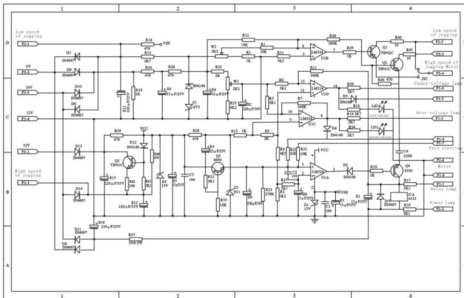
Рисунок 3: Электрическая схема
